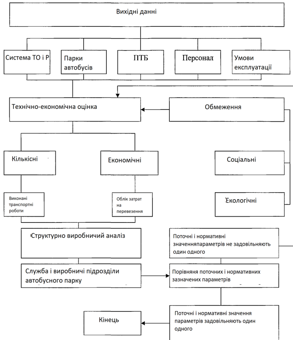
Рисунок 3.2 – Блок-схема комплексної оцінки ефективності використання міських автобусів
