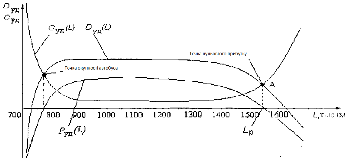
Рисунок 2.1 – Теоретична модель реалізації цільової функції визначення ресурсу міських автобусів
