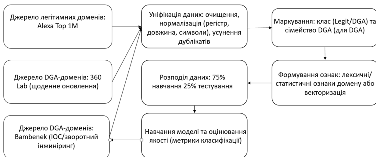
Рисунок 2.2 – Пайплайн формування набору даних для розпізнавання DGA-доменів і DGA-трафіку
