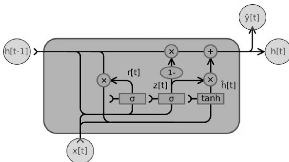
Рисунок 2.5 – Структура рекурентного блоку GRU
